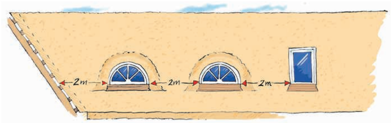
Tegning 41 Minimumsafstand mellem kviste/ovenlys/skotrende/skorsten
