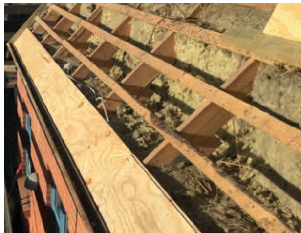
Foto 48 Vindstop ved tagfod
