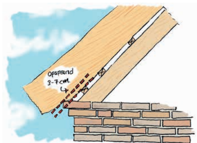
Tegning 35 Muret opspænd ved sternbræt
