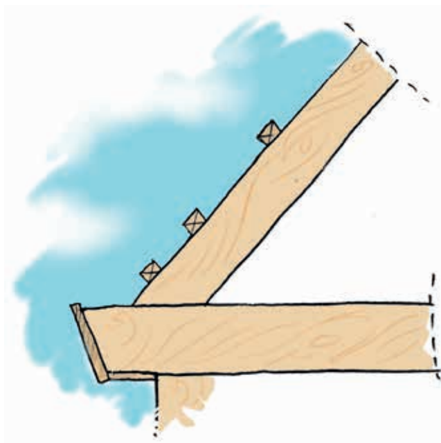
Tegning 34 Stern/sugfjæl
